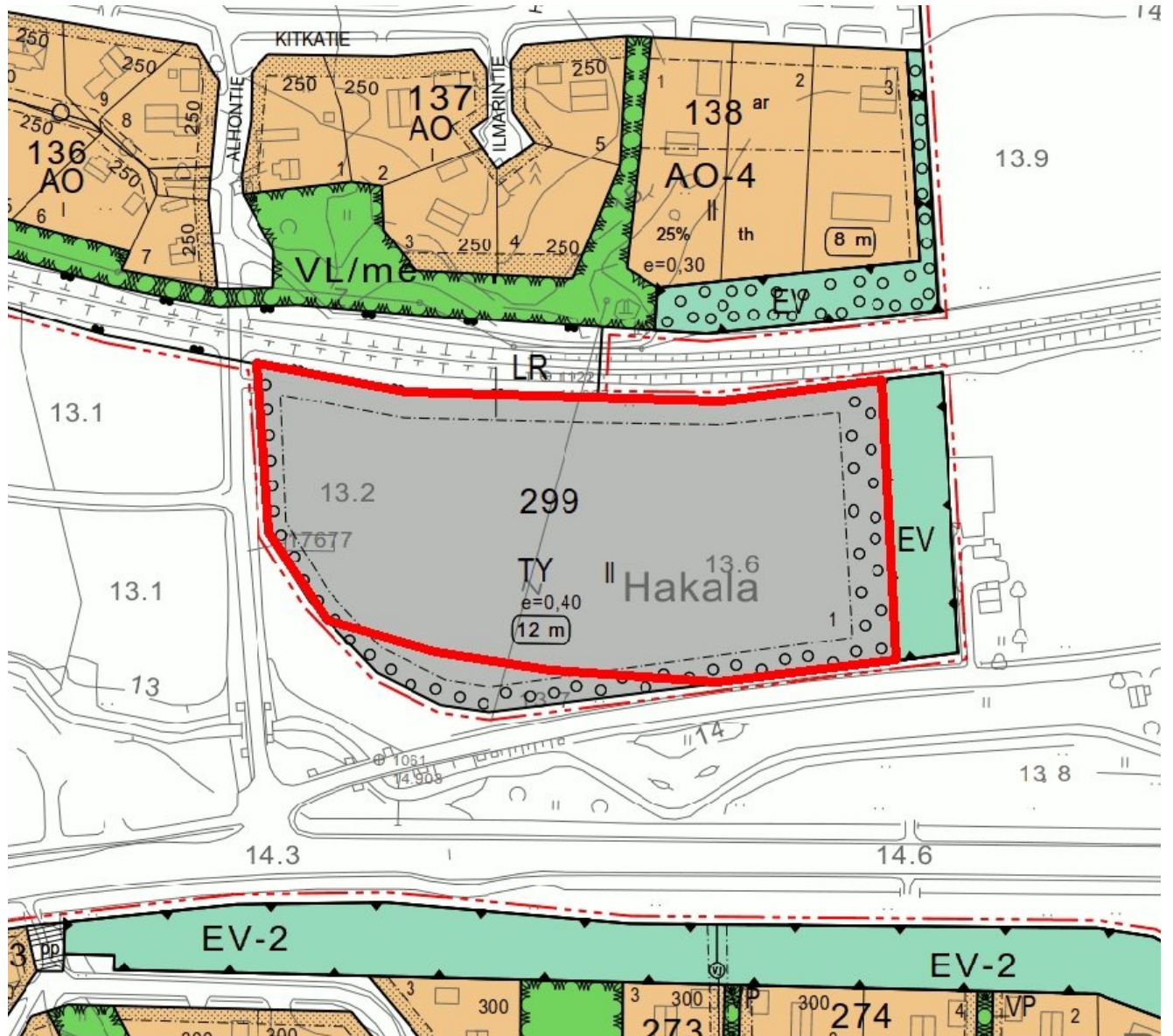
Asemakaava
